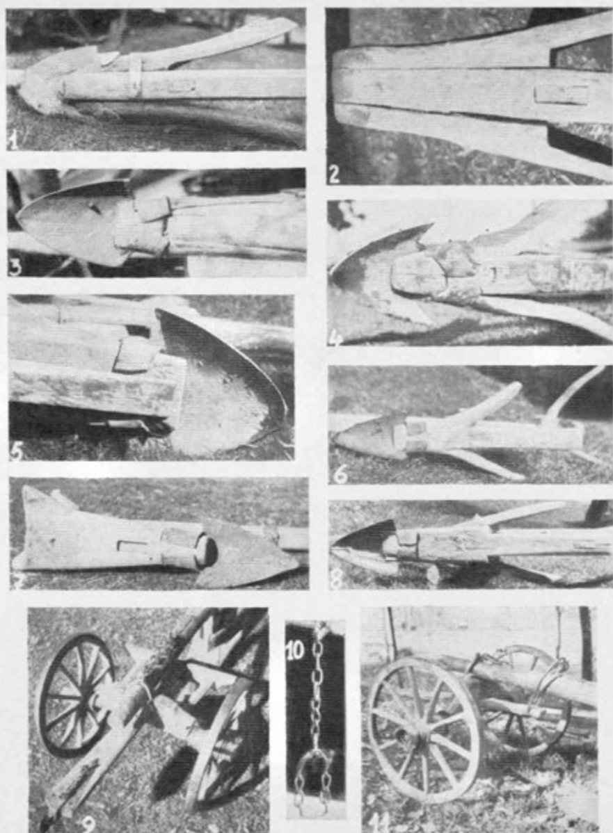
Plaz štajersko-koroškega rala z lemeškami (habami) in ralnikom ali brez njega od spodaj iz teh-le krajev: 1. St. Ilj, 2. Vovbre, 3. Vovbrske gore, 4. Rute pri Podgorju, 5. Plešivec, 6. Brezni vrh (Kobansko), 7. Sv. Križ-Sober, 8. Pernice; 9. Kolca rala z jezikom, použo in drugimi sest.deli, Dragožiče; 10. Cetna, črča (?), Pečnica pri Ledincah; 11. Kolca rala s prednjo in zadnjo gredlnico. Smarjeta v Rožu
