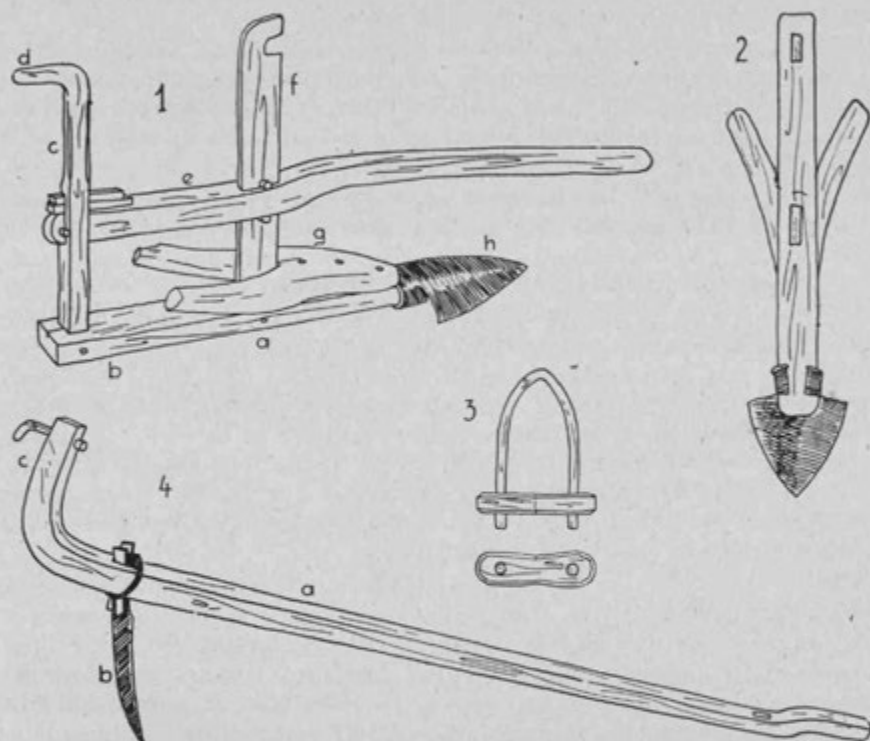
Sl. 1. Ralo iz Smihela nad Mozirjem: a podsad, b pêta, c ročica, d repac, e grédli, f kózuc, g vilce, h ralnik; 2. podsad z vilicami in ralnikom od spodaj; 3. gréglica ali grédlanca; 4. rezáunca: a uóje, b rezáunca, c držaj
