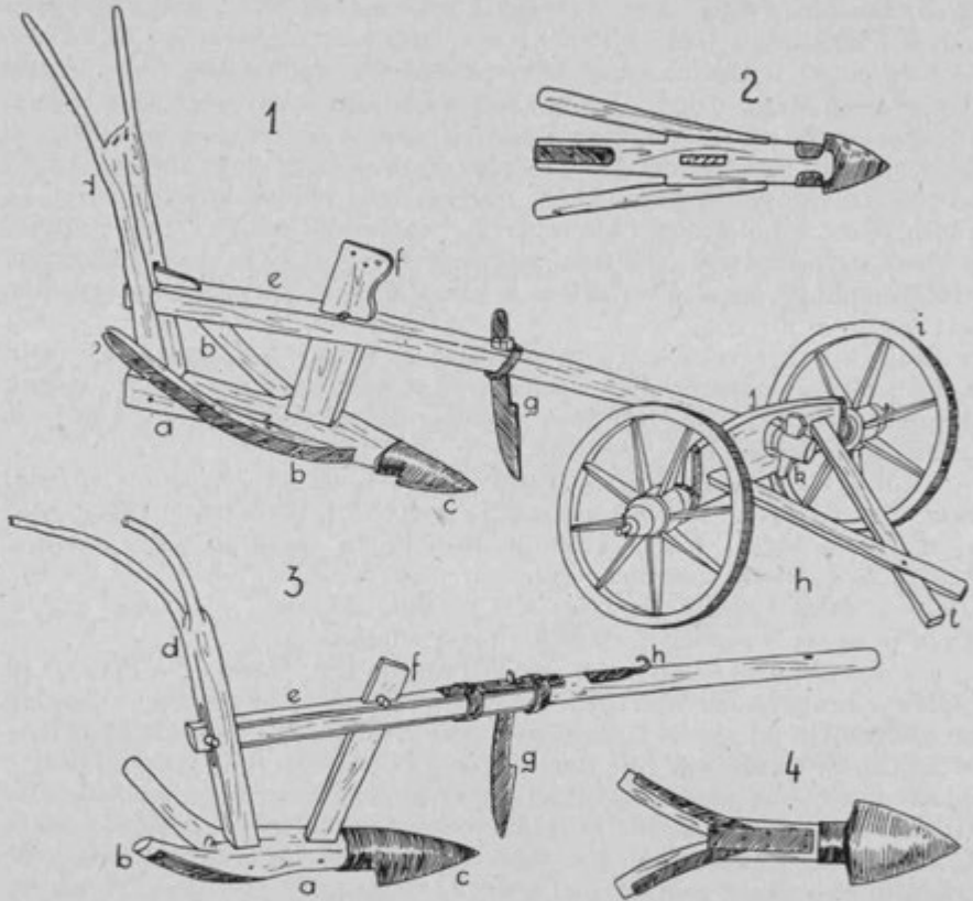
Sl. 1. Rálo iz Mlak pri Pernicah: a plát ali plátíže, b úhe, c oráunik, d pók, e grádl ali grédl, f kázuc, g rezálo, h podéuc, i kolesníce, j nóza, k žlésa; 2. plát z ušesi rala od spodaj; 3. ralo (plužnica) iz Slemena: a plóh, b rógli, c oráunik, d pók, e grédl, f žvenga, g rezánca, h hákl; 4. plaz z ušesi in ralnikom od spodaj
