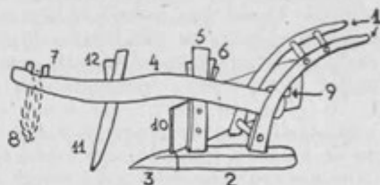
Plug. Ribno kod Bleda (točka 115 na karti). Po crtežu M. Marjanovića (1948). — 1. ručice (ročice); 2. plaz (posad); 3. lemeš; 4. gredelj (gredel, greben); 5. kozlaci (domaći naziv nije zabilježen); 6. klin; 7. kurelj (prikav); 8. gredeljnica (bradanca); 9. zagušnjak (zagojzda); 10. daska (deska, dila); 11. crtalo (črtov) i 12. klin
