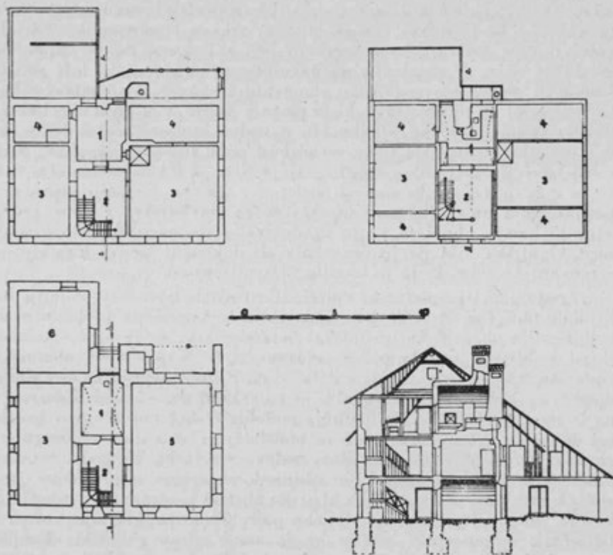
Sl. 1. Obrtniška (Šepetavčeva) rudarska hiša v Idriji (1 kuhinja, 2 lopa, 3 rodbinske sobe, 4 sobe za goste, 5 delavnica, 6 klet); posnel 1955 lv. Jereb.
